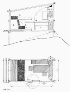
166. Coupe et plan du refuge Bivouac. Dessin Charlotte Perriand, André Tournon, ingénieur, 1936. AChP - Charlotte Perriand © ADAGP, Paris 2016
